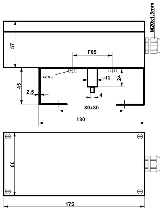
dimensions
