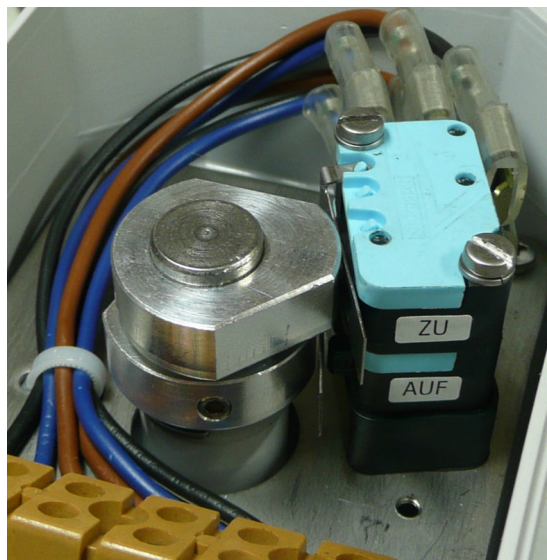
Abb.: Innenansicht der mechn. Crouzet V3-Endschalter mit verstellbaren Schaltnocken 0 - 180°
