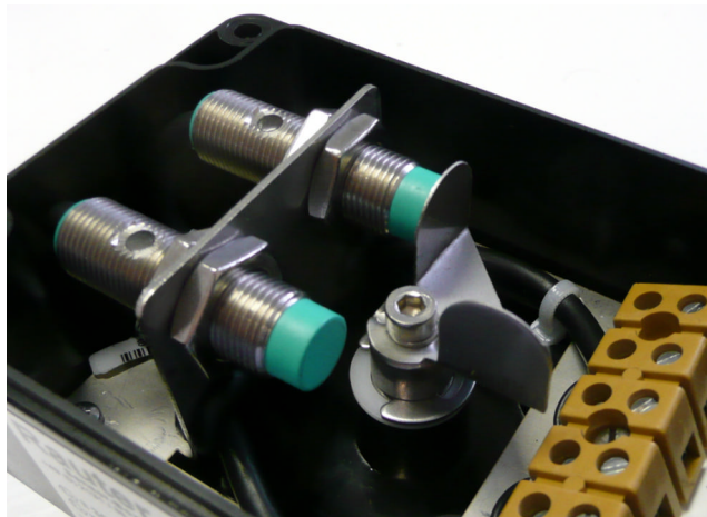
Abb.: Innenansicht der Pepperl+Fuchs Sensoren NJ-12GM40-E2 mit LED und 0 und 90° Schaltfahne
