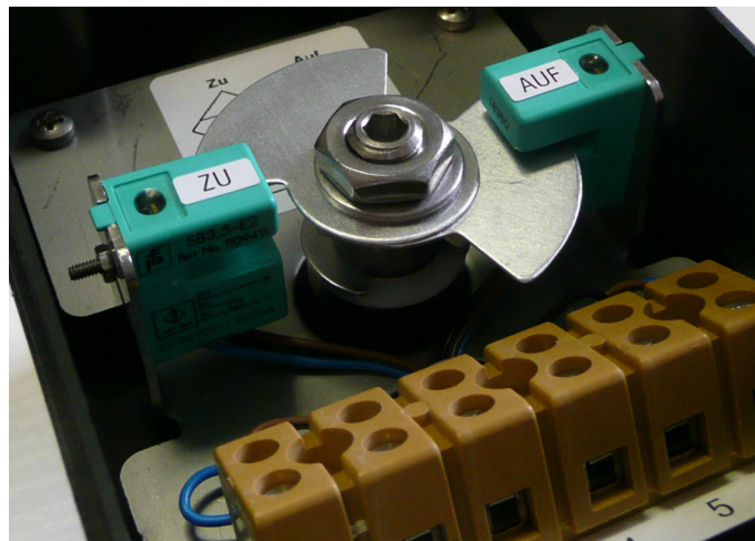
Abb.: Innenansicht der Pepperl+Fuchs Sensoren SB 3,5-E2 mit separat verstellbaren Schaltfahnen
