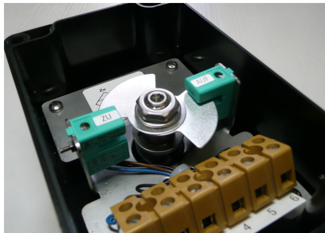
Abb.: Innenansicht der Pepperl+Fuchs Sensoren SB 3,5-E2 mit LED und separat einstellbaren Schaltfahnen
