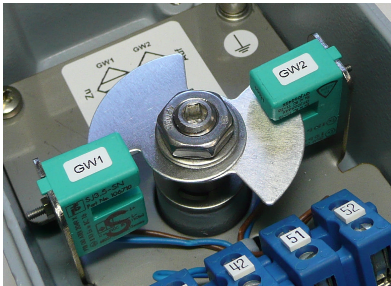
Abb.: Innenansicht der Pepperl+Fuchs - 45°C Schlitz-Sensoren SJ 3,5-SN mit separat einstellbaren Schaltfahnen
